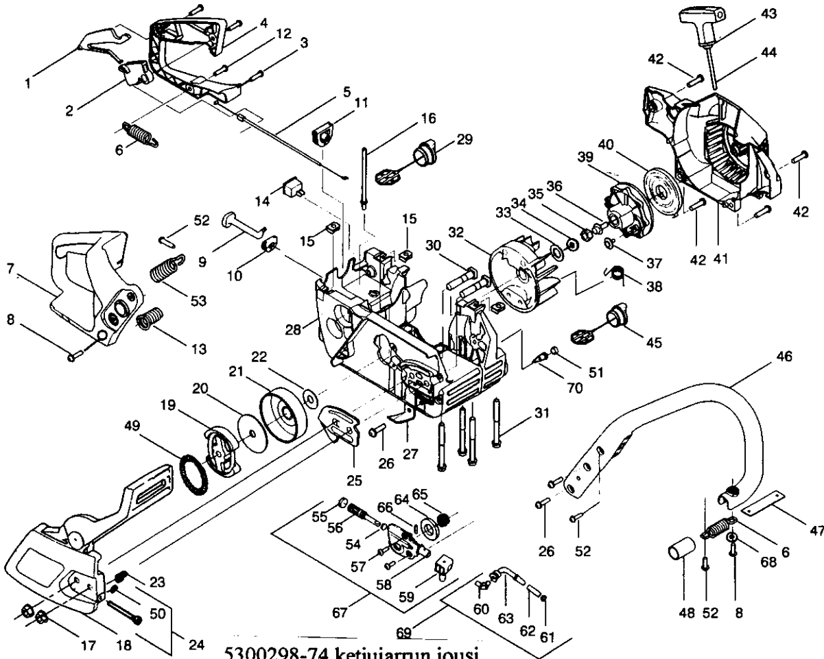
5300298-74 ketjujarrun jousi
